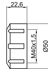
Nut GT 32
